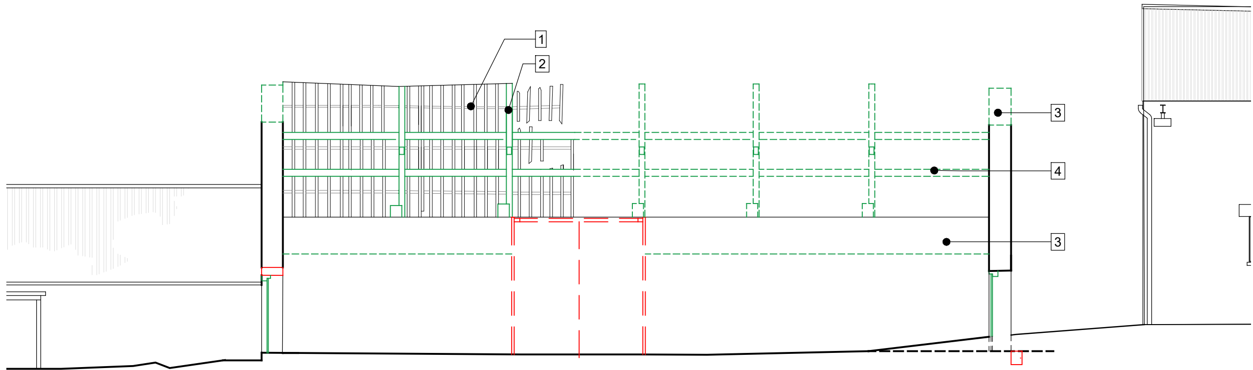
1 Long Section 5100 1:100
